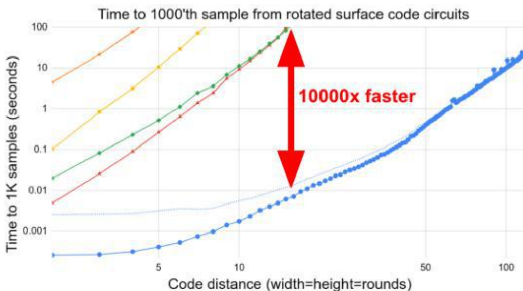
图 27 在稳定器电路的批量采样方面，Stim 明显快于以前的工具
