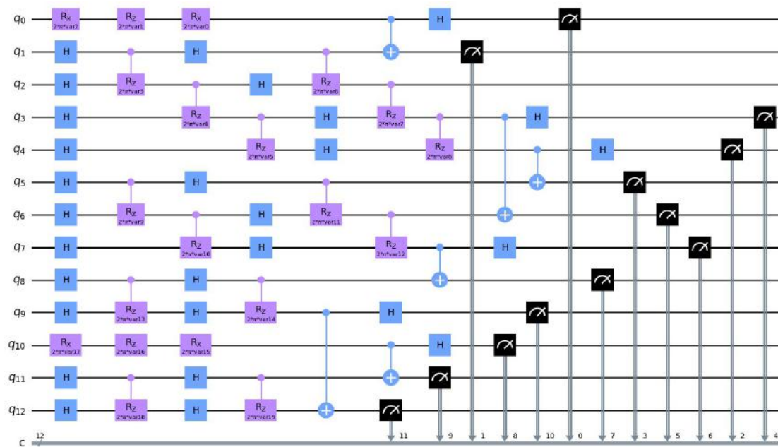
图 21 lambeq 将句子转换成量子电路
