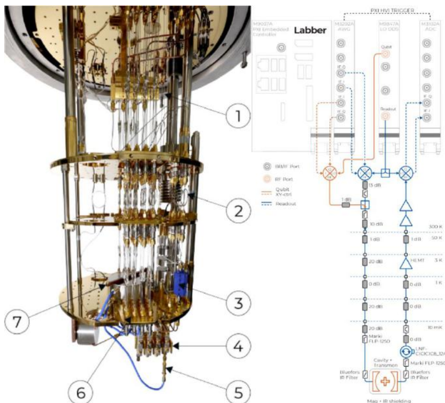
图 7 是德科技集成测控系统。左图是 Bluefors LD250 稀释制冷机；右图是量子测控系统与稀释制冷机的集成
