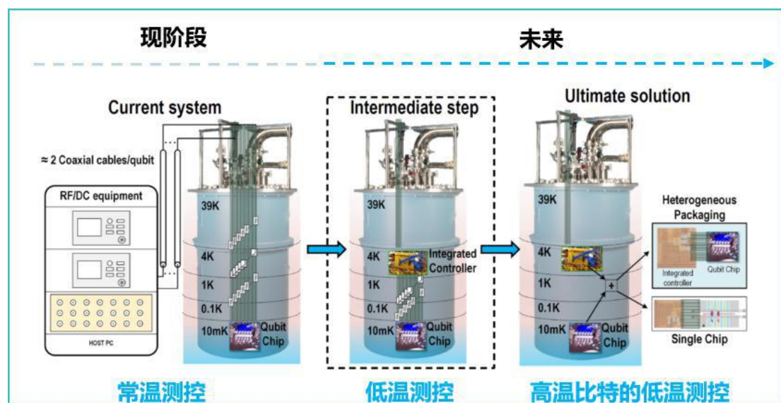
图 4 量子计算测控系统发展趋势
