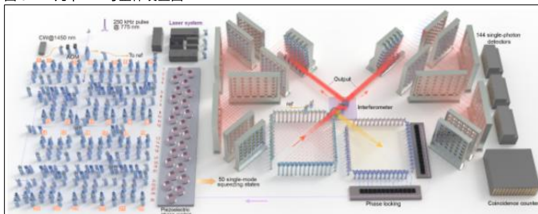
图 31 “九章”二号整体装置图
