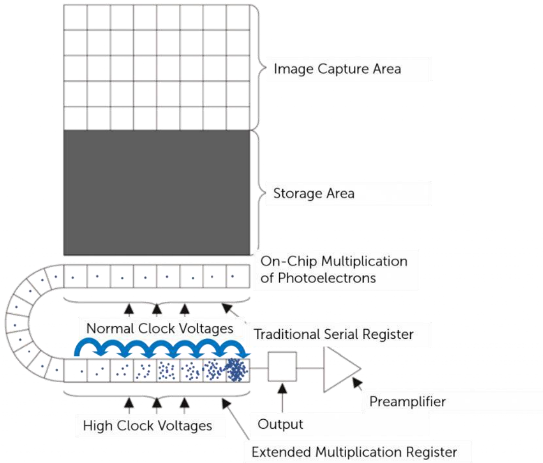
图 15 EMCCD 芯片结构图
