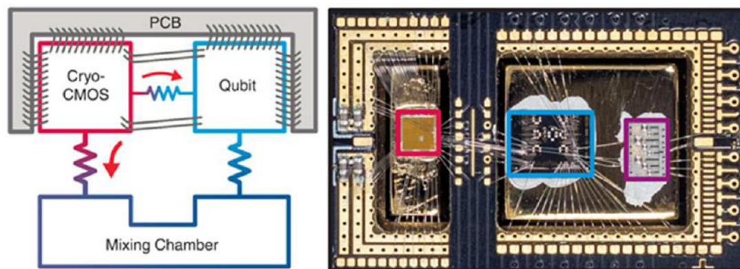
图 28 微软低温控制芯片 Gooseberry
