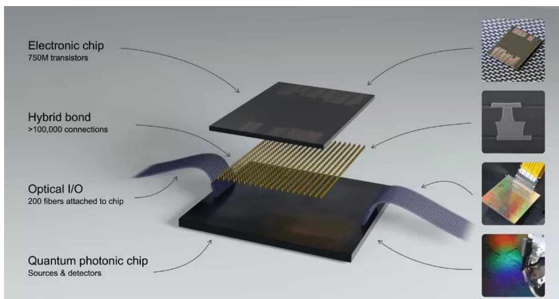
图 30 PsiQuantum 光量子芯片
