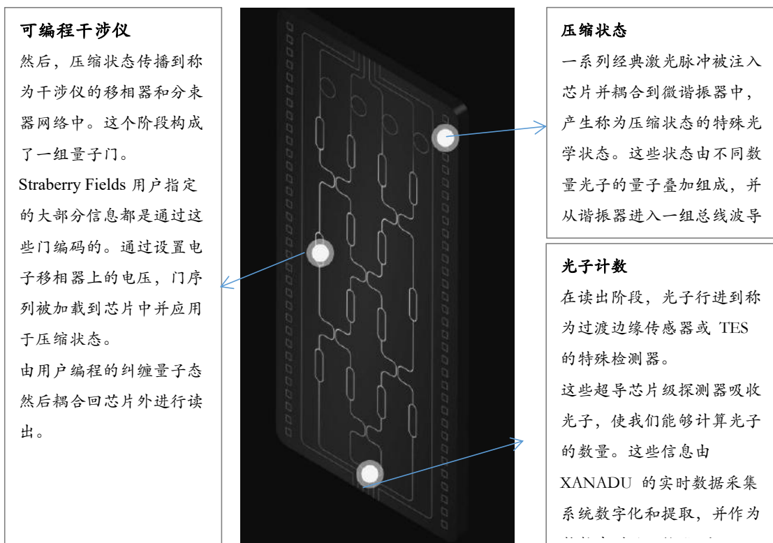
图 29 Xanadu 可编程光量子芯片
