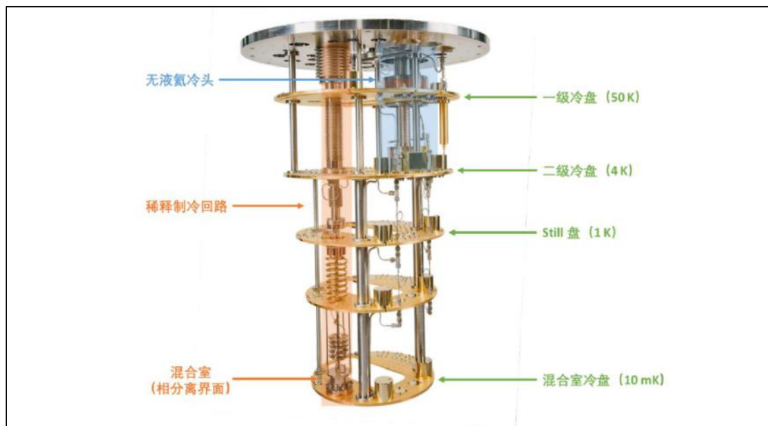
图 2 稀释制冷机内部结构
